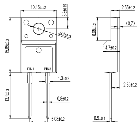
ITO-220AC DR20XXF
